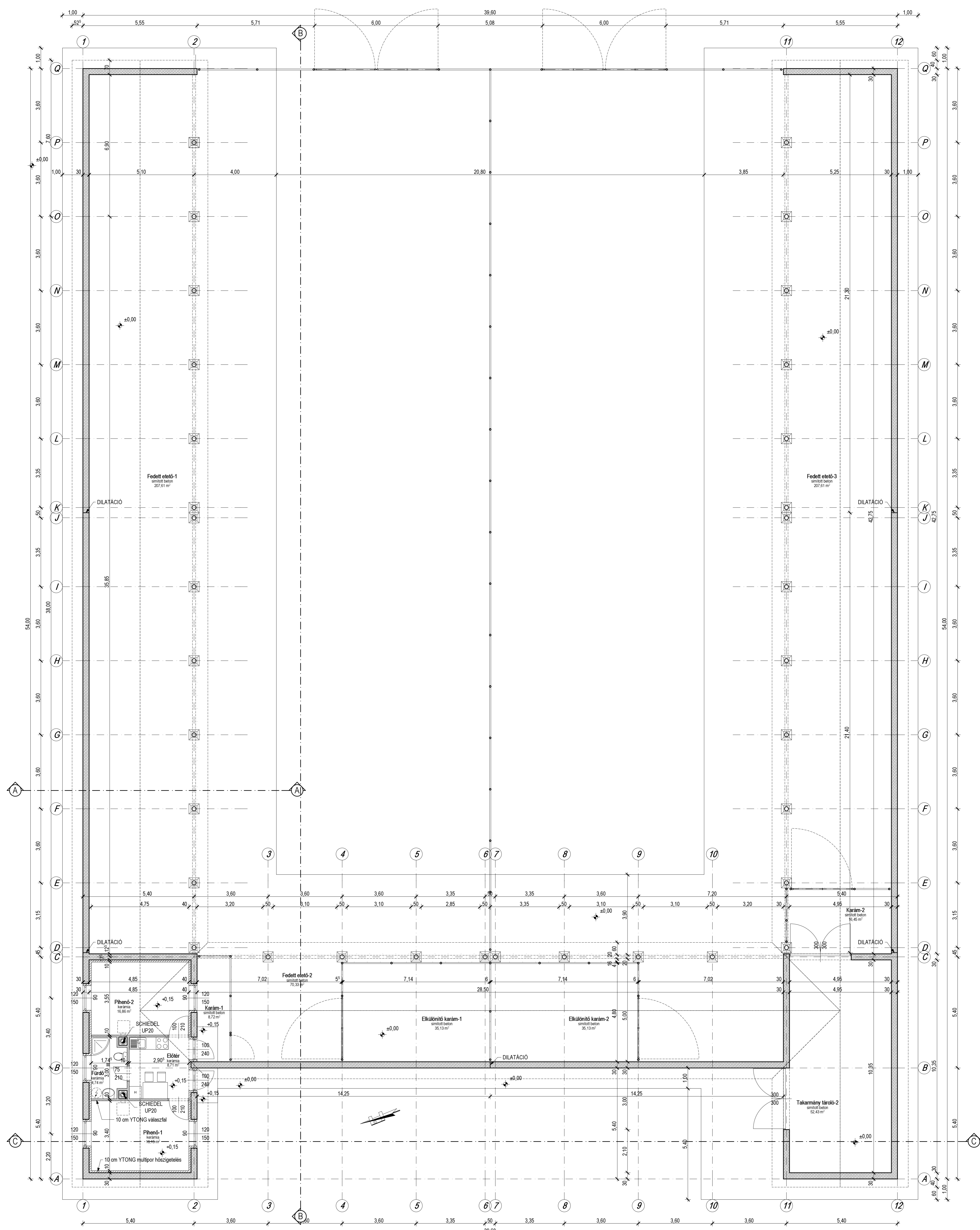
ALAPRAJZ M 1:100
